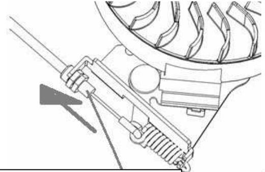
KOPPELINGSKABEL -AFSTELLING
